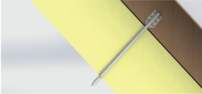
1. Fixer la suspente sur la charpente
